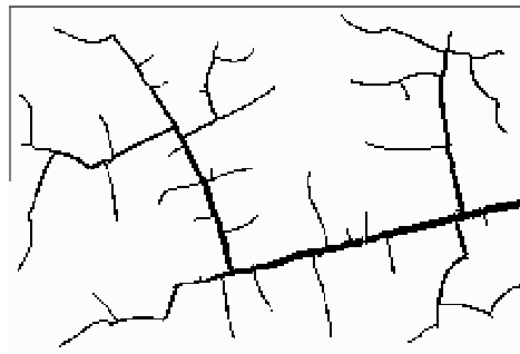
(d) n = 54 , \gamma = -3.5 , \beta = -5 \cdot 10^{-7}
